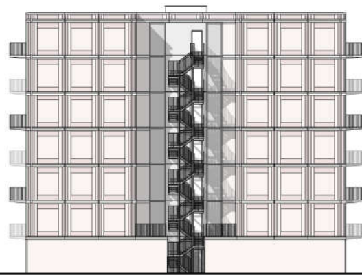
Gevelaanzicht Noord North Elevation
