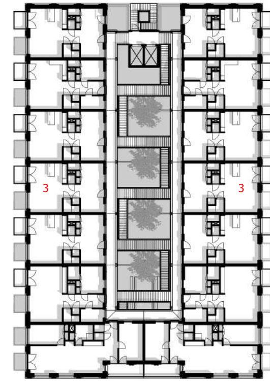
2e t/m 6e Verdieping Second up to Sixth Floor
