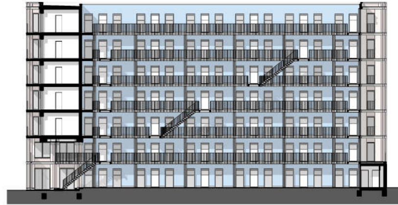
Langsdoorsnede Longitudinal Section
